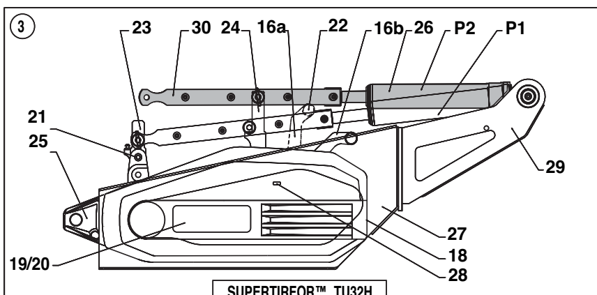
SUPERTIRFOR™ TU32H
