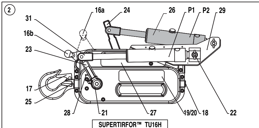
SUPERTIRFOR™ TU16H
